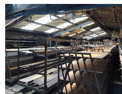
焼成窯の排気熱を利用した乾燥室
