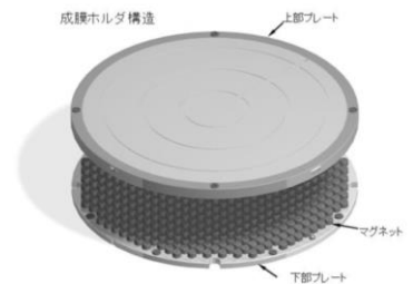
成膜ホルダ構造 (株)システム技研
